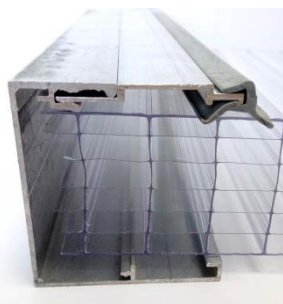
Профиль рамный для 40 мм (U, S) арт. 420040
