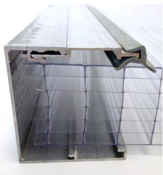
U-коннектор (ПК) арт. 380061
